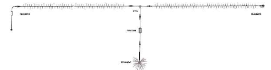
▶ Schéma de principe H558WFX - FCL080G-E - Montage en traversée
